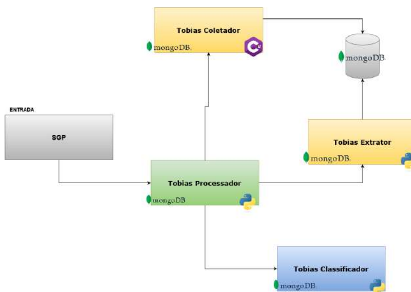
Imagem 2 - Arquitetura de Tobias 2.0
